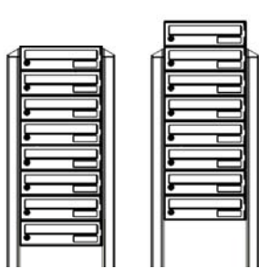
Az ábra a 8 egységből álló rendszer szerelését ábrázolja (Terzo talp és bebetonozva)
