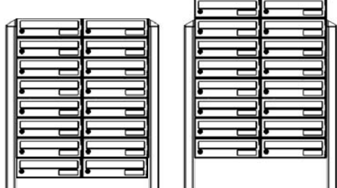
Az ábra a 16 egységből álló rendszer szerelését ábrázolja (Terzo talp és bebetonozva)
